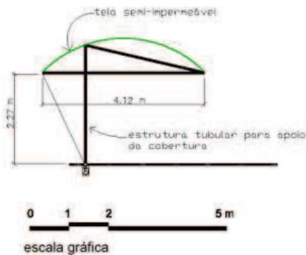
Corte esquemático
