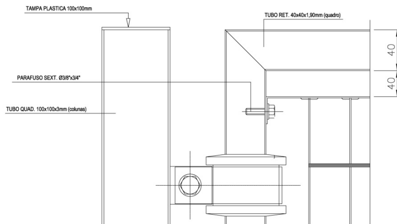
DETALHE-B
