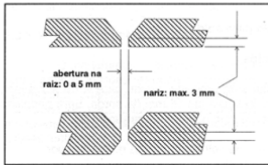
Figura 1 – Tolerâncias dimensionais
