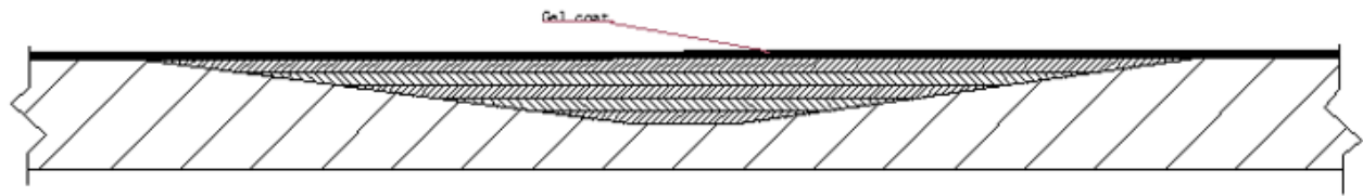
Reparo em dano parcial na espessura
