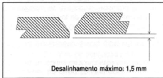
Figura 3 – Desalinhamento máximo
