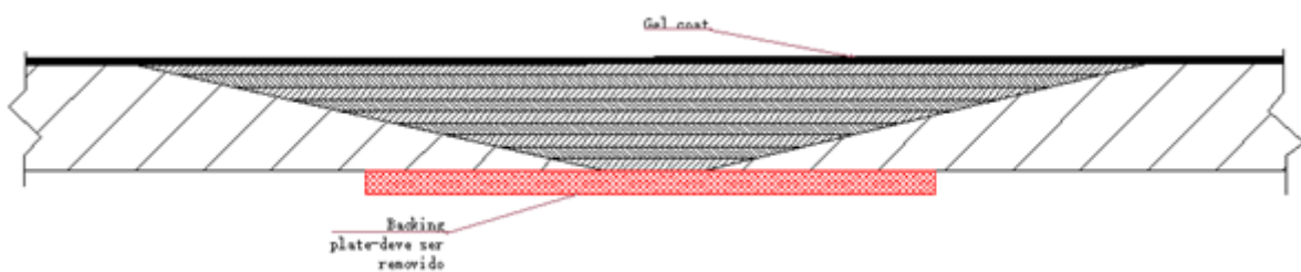
Reparo em dano em toda a espessura com chanfro simples
