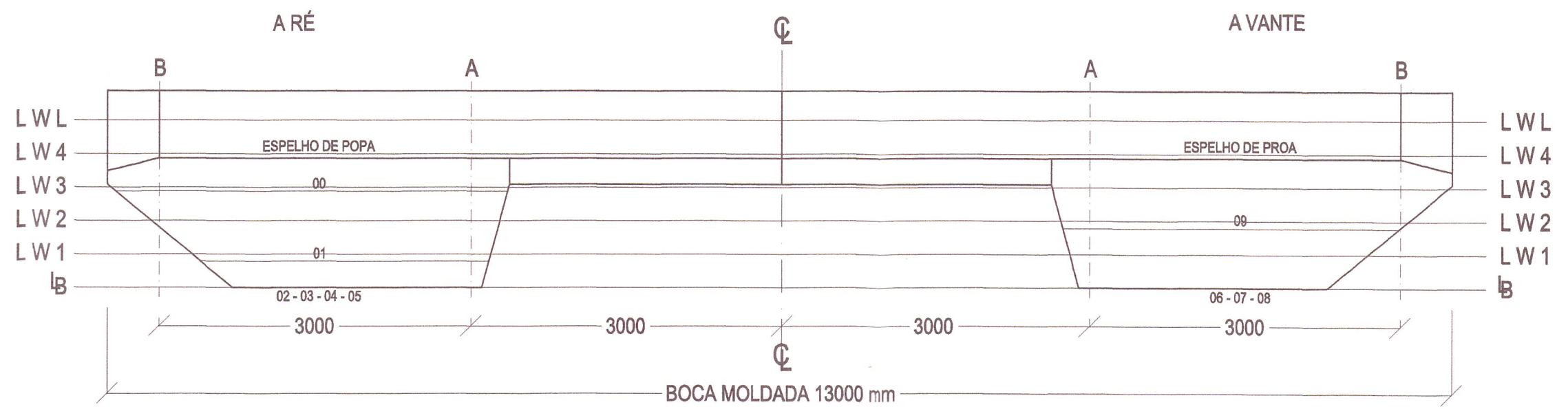
PLANO DE BALIZAS
