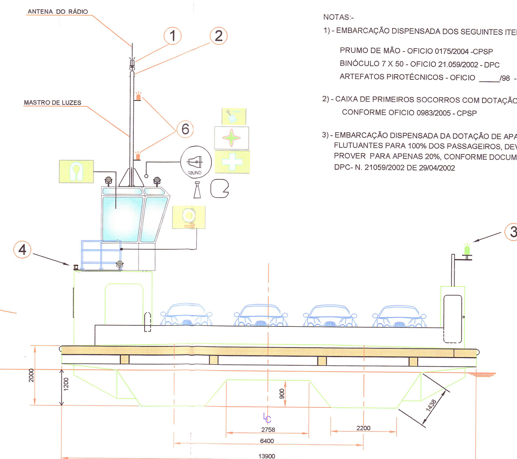
SEÇÃO TRANSVERSAL
