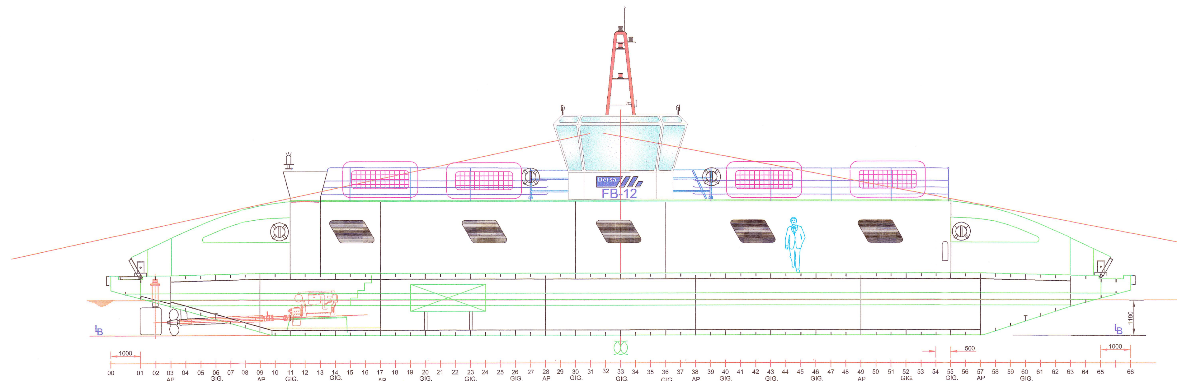
PERFIL LONGITUDINAL Á 3200 DA L.C.
