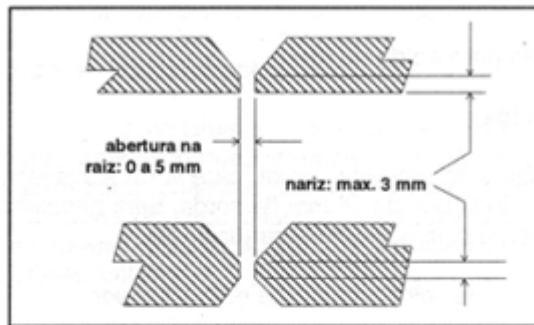
Figura 1 – Tolerâncias dimensionais
