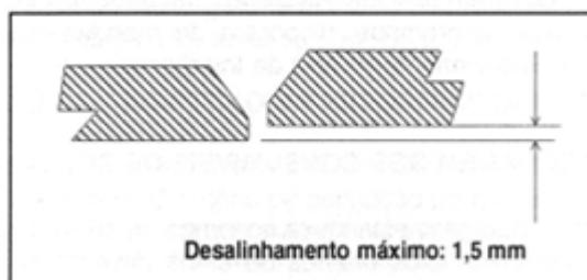
Figura 3 – Desalinhamento máximo
