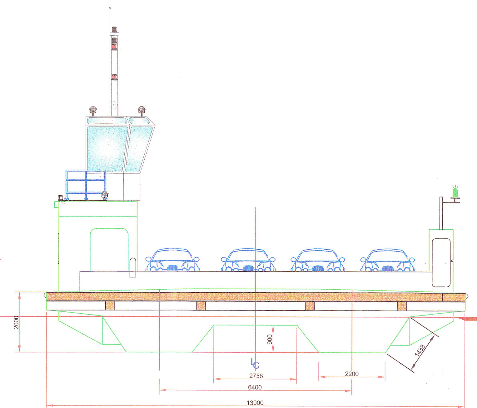
SEÇÃO TRANSVERSAL
