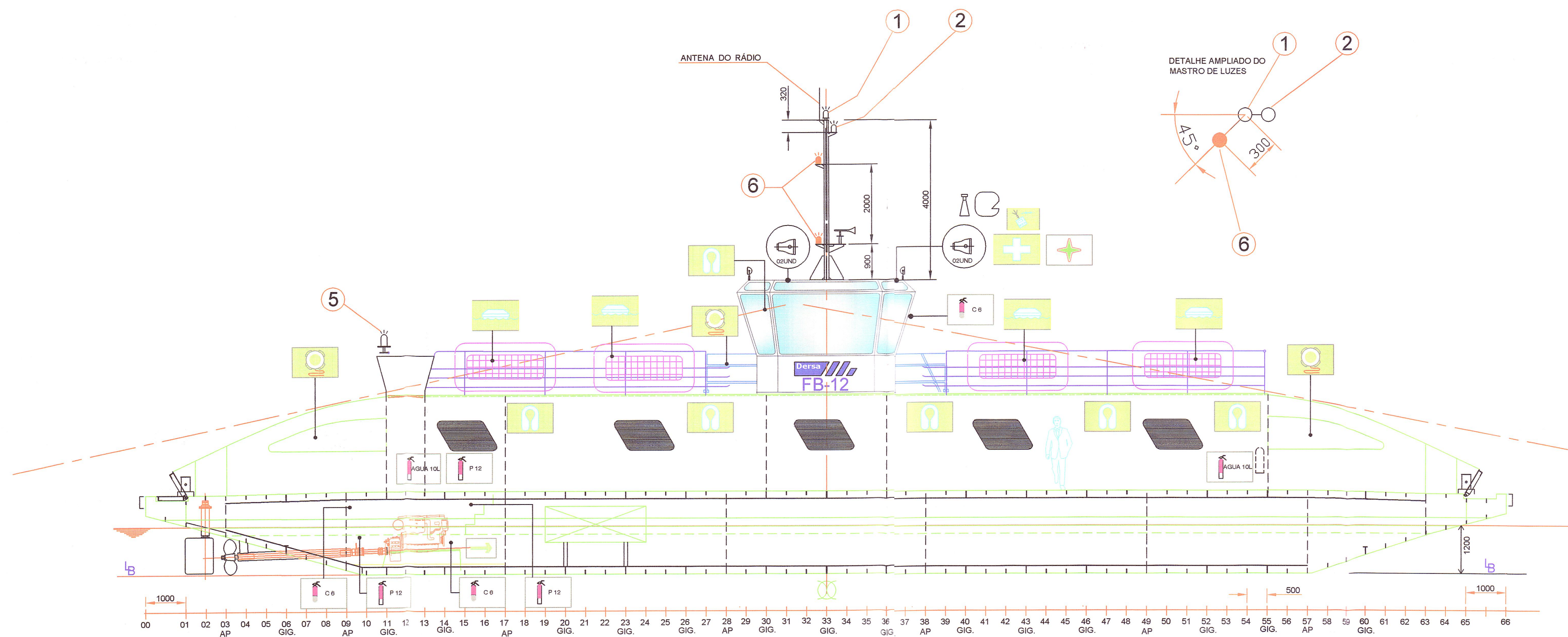
PERFIL LONGITUDINAL Á 3200 DA L.C.
