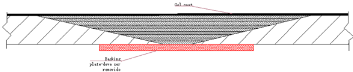
Reparo em dano em toda a espessura com chanfro simples
