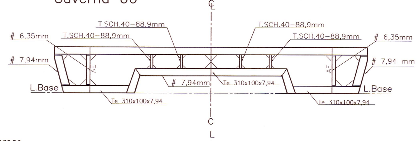
SEÇÃO TRANSVERSAL Caverna 06
