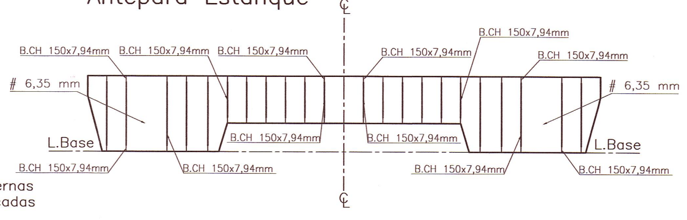
SEÇÃO TRANSVERSAL Antepara Estanque
