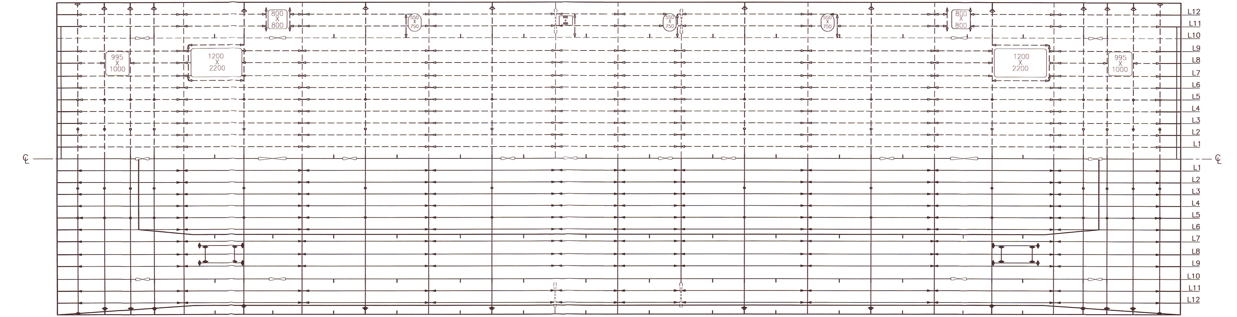
VISTA DO CONVÉS
