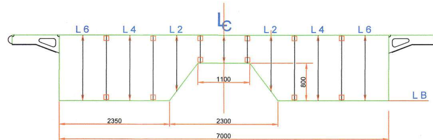
SEÇÃO DAS ANTEPARAS NAS CAV. 6 E 44
