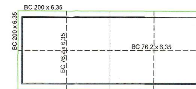
VISTA DO CONVÉS DO TIJUPÁ
