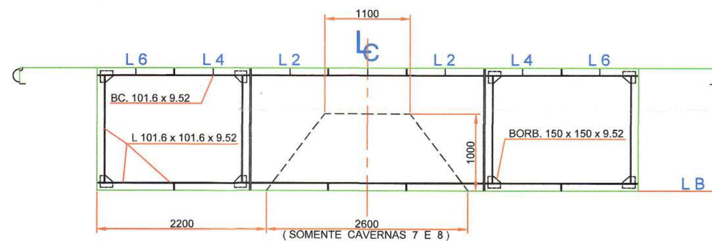
SEÇÃO DAS CAVERNAS COMUNS
