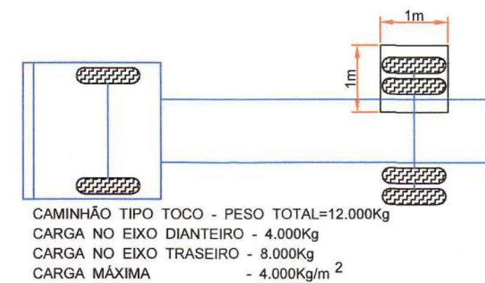
CARGA DE PROJETO PARA O CONVÉS
