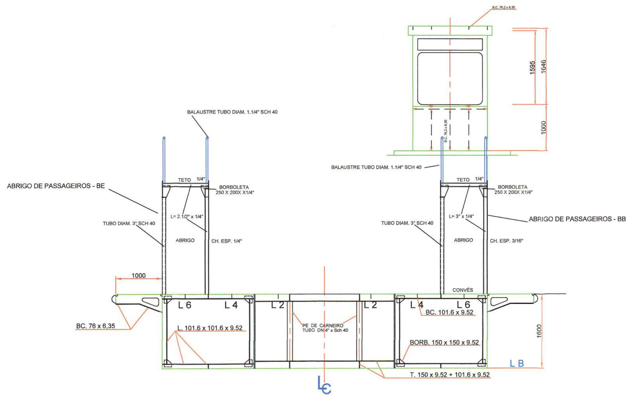
SEÇÃO DAS CAVERNAS 22 E 28
