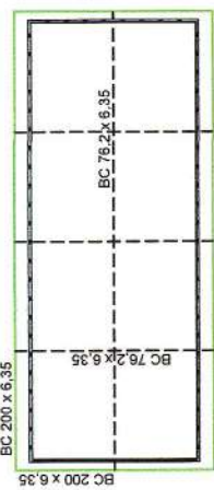
VISTA DO CONVÉS DO TIJUPA
