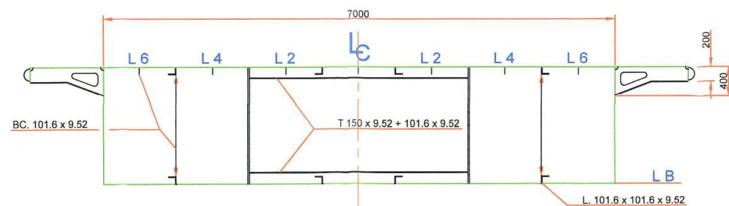
SEÇÃO DAS CAVERNAS 18 E 32
