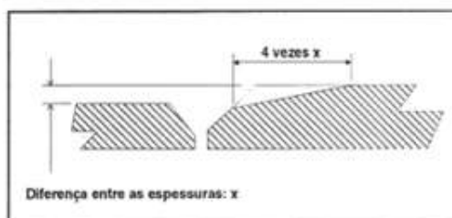
Figura 4 – Correção para x \geq 3 \text{ mm}
