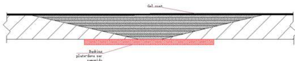
Reparo em dano em toda espessura com chanfro simples
