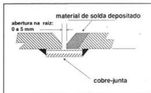
Figura 2 – Correção de abertura excessiva
