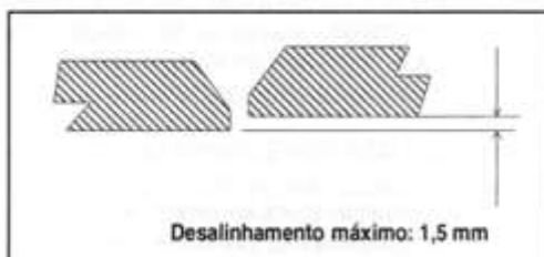
Figura 3 – Desalinhamento máximo
