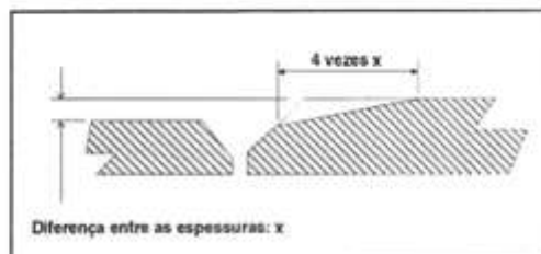
Figura 4 – Correção para x \geq 3 mm
