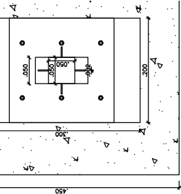
planta placa 0,30m x 0,20m escala 1:10
