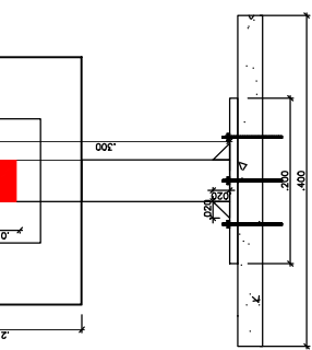
elevação placa 0,30m x 0,20m escala 1:10
